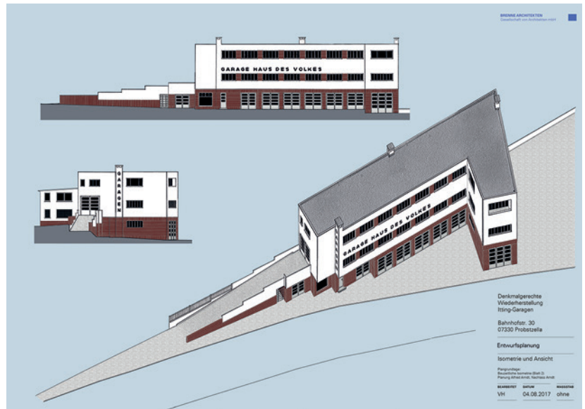
Probstzella: Isometrie und Ansicht der Itting-Garagen
