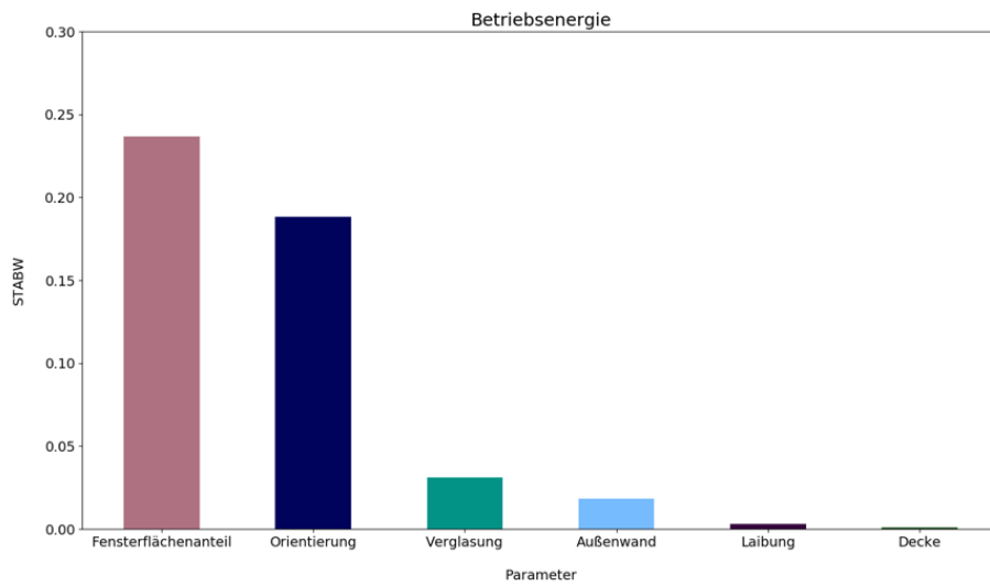
Abbildung 57_Ranking der einzelnen passiven Parameter Betriebsenergie (Eigene Darstellung)
