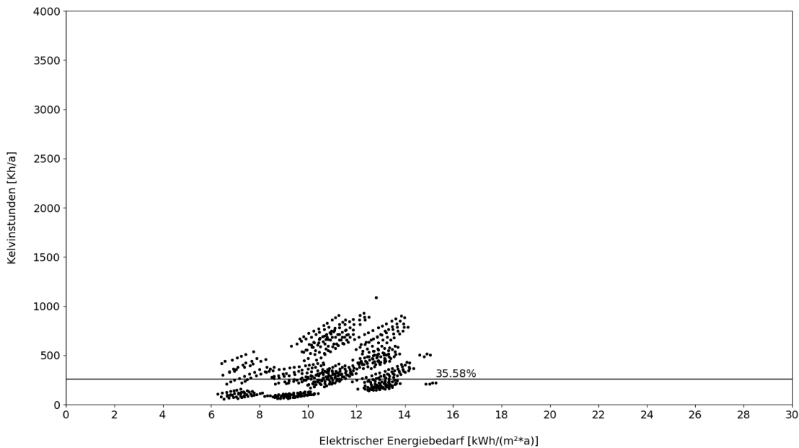
Abbildung 30_ Punktwolke der Ergebnisse passiv++ ergänzendes System Sonnenschutz (Eigene Darstellung: Therm. Simulation)
