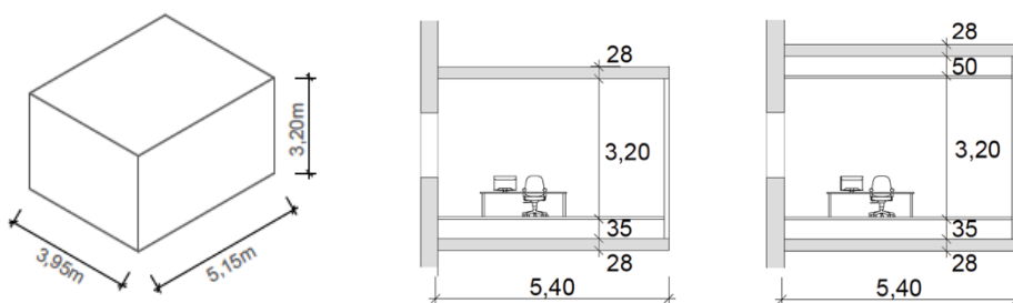
Abbildung 10 a-c_Raumvolumen + lichte Raummaß (Eigene Darstellung)
