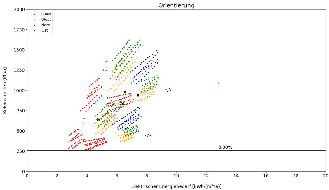
Abbildung 51_Parameter Orientierung - passiv ++ Sonnenschutz_SEMINAR (Eigene Darstellung: Therm. Simulation)
