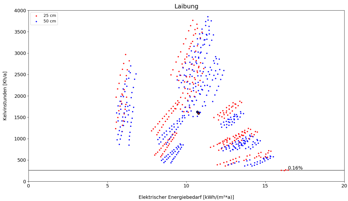
Abbildung 28_ Parameter Eigenverschattung / Laibung Innenausbau - passiv+ (Eigene Darstellung: Therm. Simulation)
