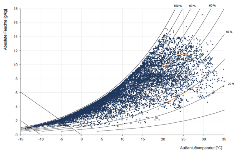
Abbildung 8_hx Diagramm (Eigene Darstellung: Therm. Simulation)
