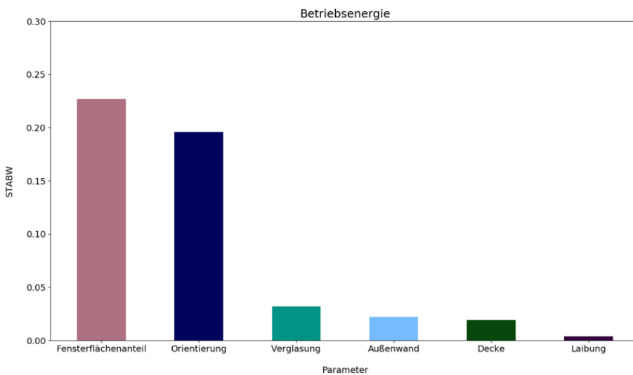
Abbildung 55_Ranking der einzelnen passiven Parameter Betriebsenergie (Eigene Darstellung)
