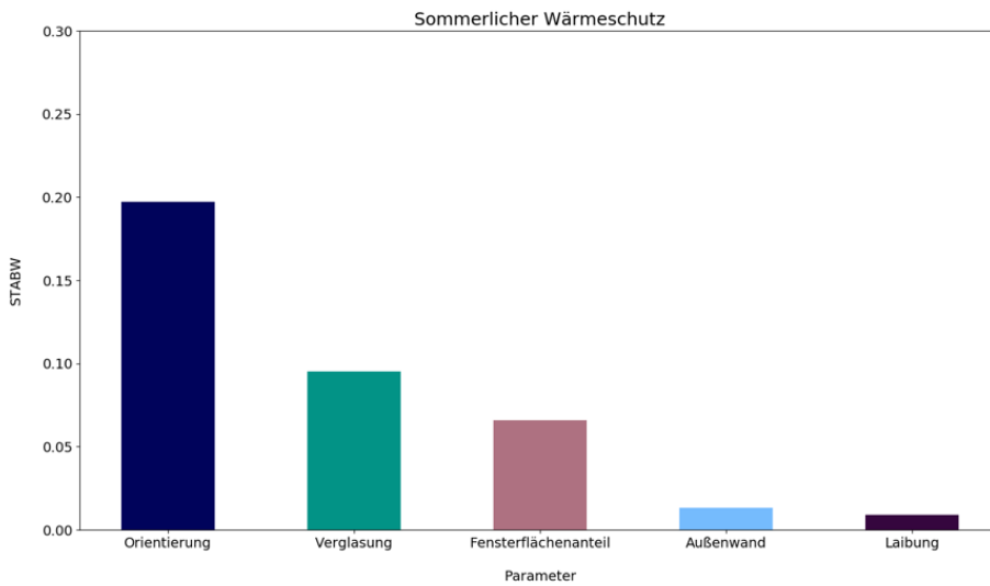
Abbildung 60_Ranking der einzelnen passiven Parameter sommerliches Verhalten (Eigene Darstellung)
