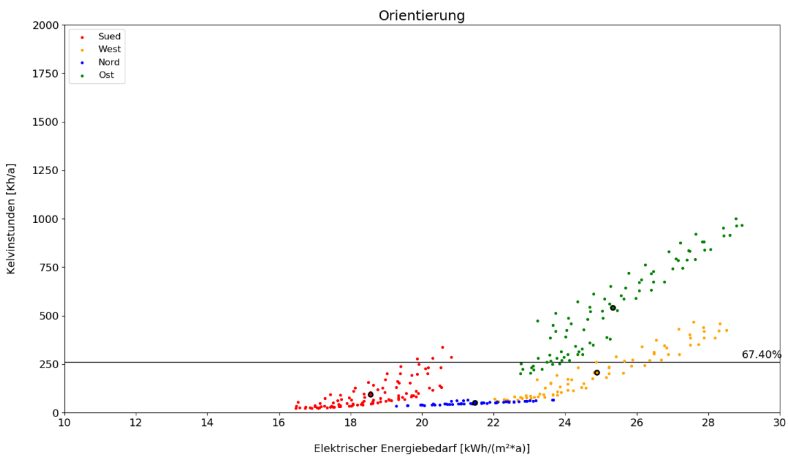
Abbildung 45_Parameter Orientierung - passiv++ BKT(Eigene Darstellung: Therm. Simulation)
