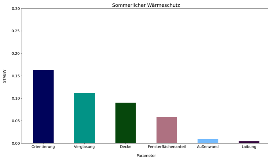
Abbildung 54_Ranking der einzelnen passiven Parameter sommerliches Verhalten (Eigene Darstellung)
