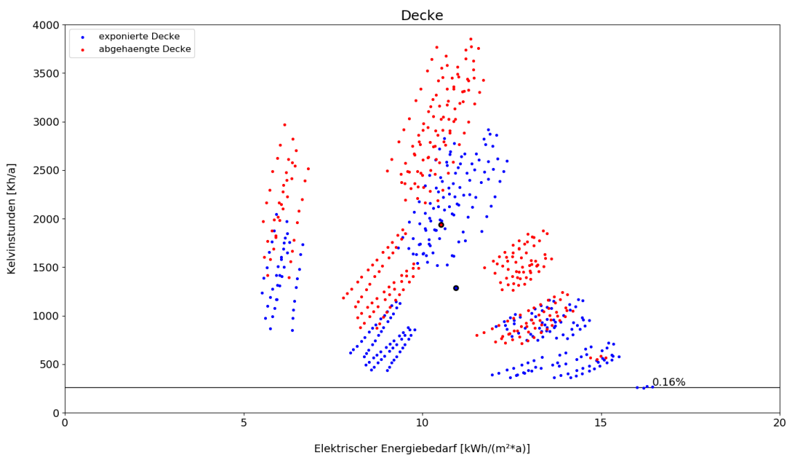
Abbildung 29_ Parameter Anteil wirksame thermische Speichermassen Decke - passiv+ (Eigene Darstellung: Therm. Simulation)
