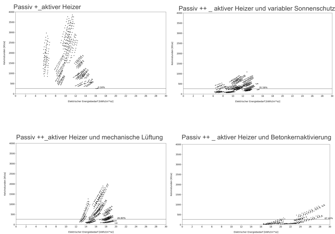
Abbildung 50_Übersicht Punktwolken der unterschiedlichen Randbedingungen passiv + und passiv ++ (Eigene Darstellung: Therm. Simulation)
