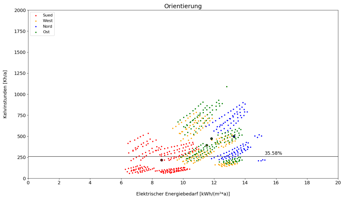
Abbildung 31_ Parameter Orientierung - passiv++ Sonnenschutz (Eigene Darstellung: Therm. Simulation)
