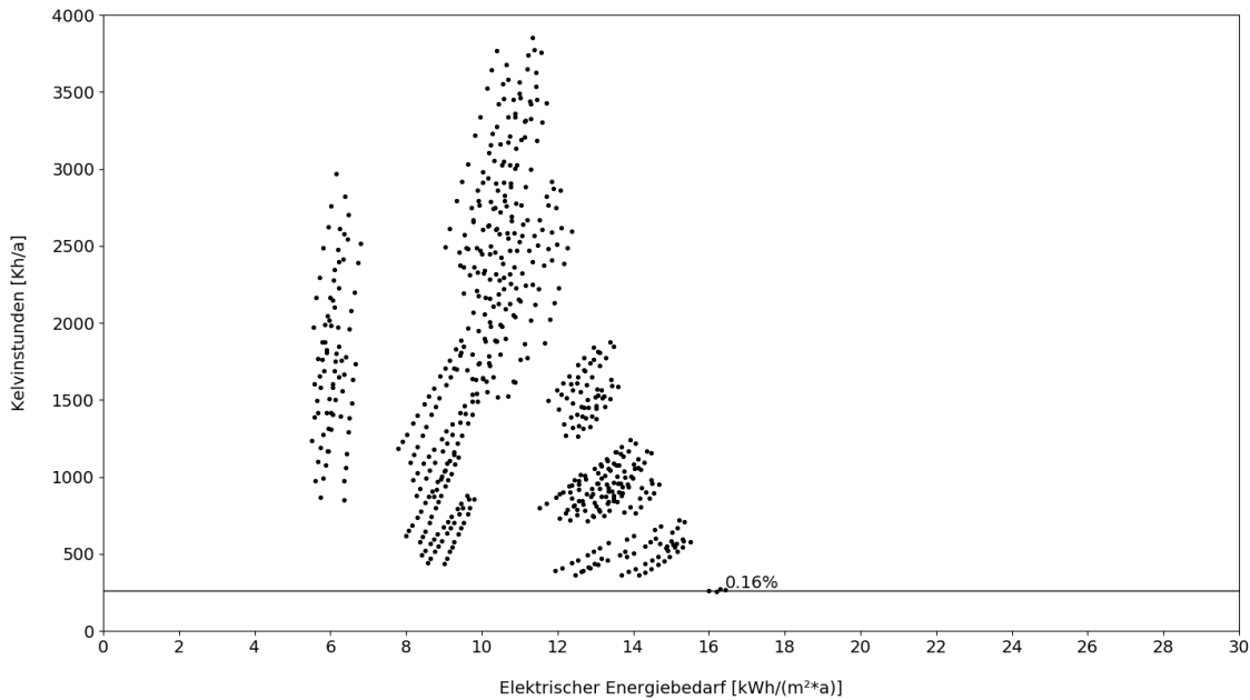
Abbildung 23_Punktwolke der Ergebnisse passiv+ (Eigene Darstellung: Therm. Simulation)
