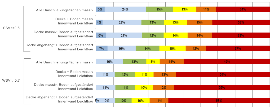
Abbildung 17_ Verteilung operative Temperaturen_Lüftungsszenario 2 + CO 2 (Eigene Darstellung)
