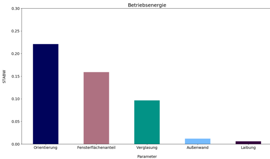
Abbildung 61_Ranking der einzelnen passiven Parameter Betriebsenergie (Eigene Darstellung)
