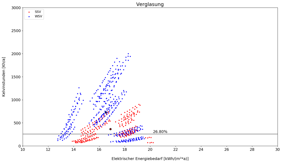
Abbildung 40_Parameter Glasqualität - passiv++ mech. Lüftung (Eigene Darstellung: Therm. Simulation)
