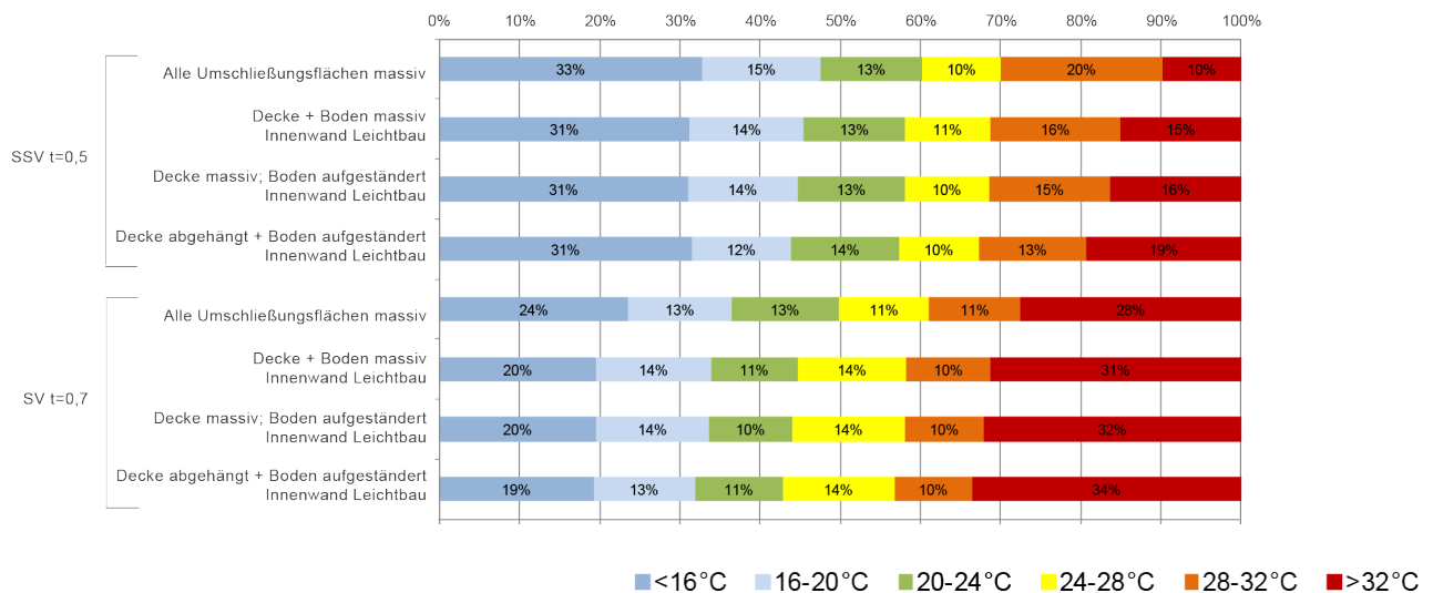
Abbildung 16_Verteilung operative Temperaturen_Lüftungsszenario 1 (Eigene Darstellung)
