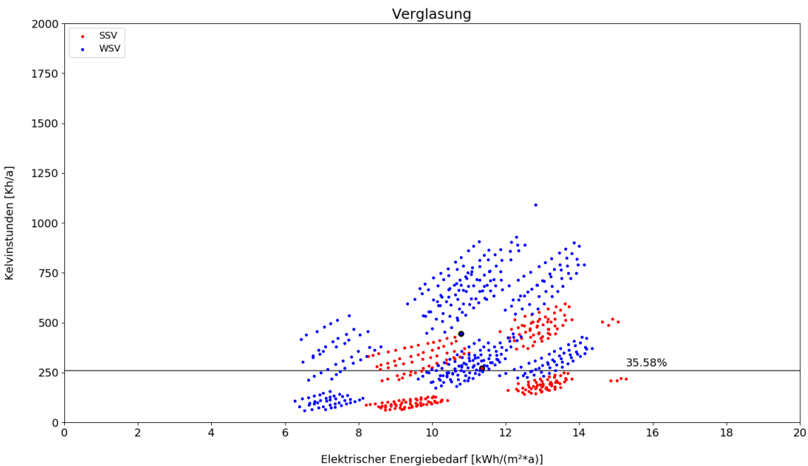
Abbildung 33_Parameter Verglasung - passiv++ Sonnenschutz (Eigene Darstellung: Therm. Simulation)
