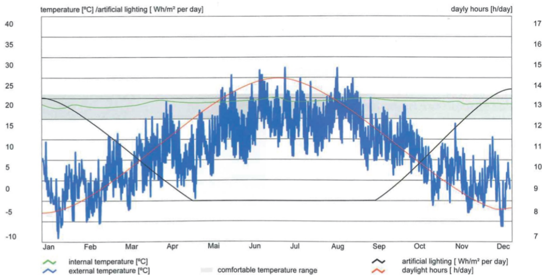
Abbildung 3_Jahresverlauf Außen- und Innenraumtemperatur Gebäude 2226 (Eigene Darstellung)
