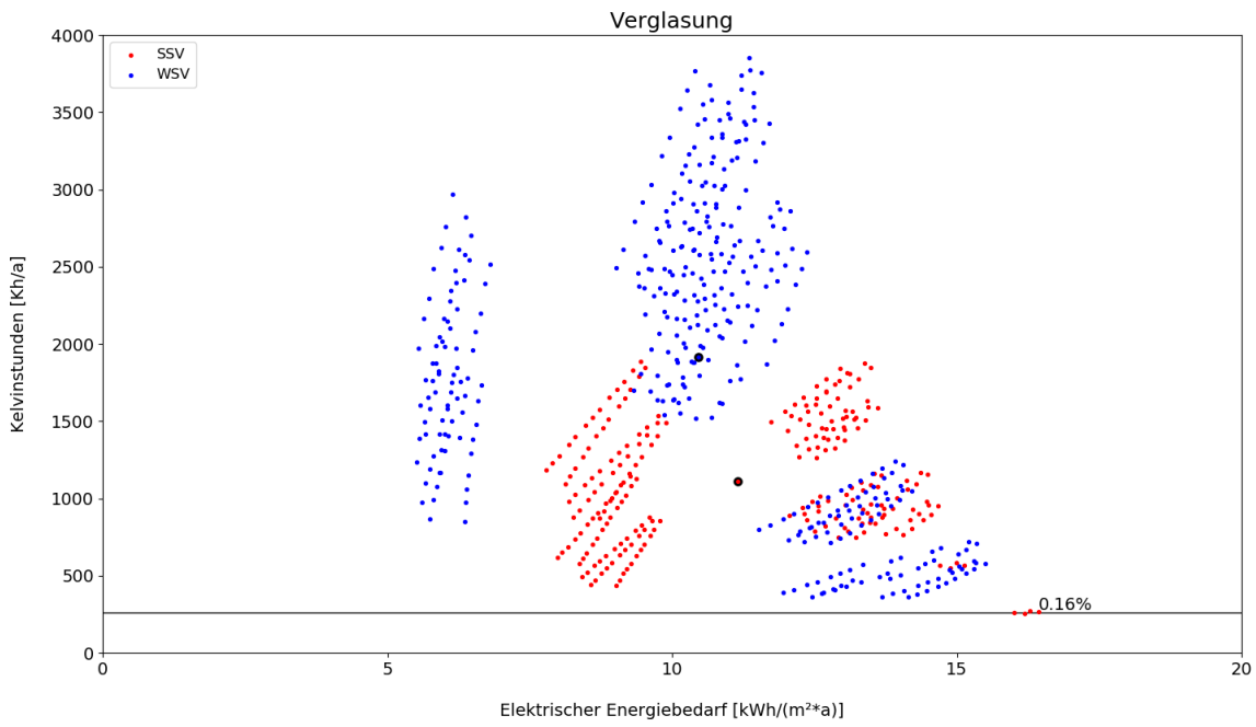
Abbildung 26_Parameter Glasqualität / Verglasung WSV – SSV - passiv+ (Eigene Darstellung: Therm. Simulation)
