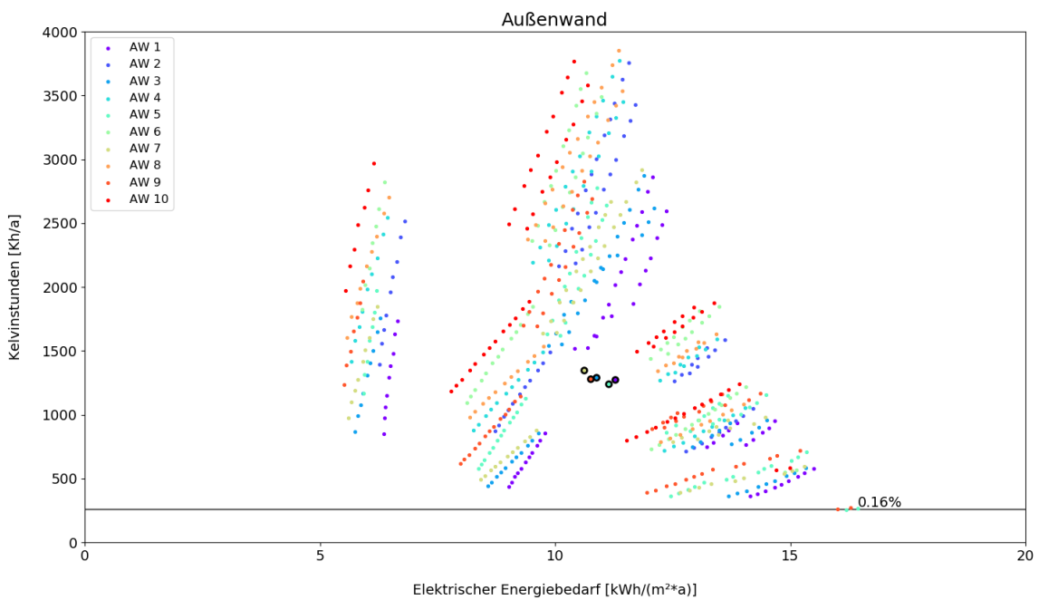
Abbildung 27_Parameter Baukonstruktion AW + thermische Masse Innenausbau - passiv+ (Eigene Darstellung: Therm. Simulation)
