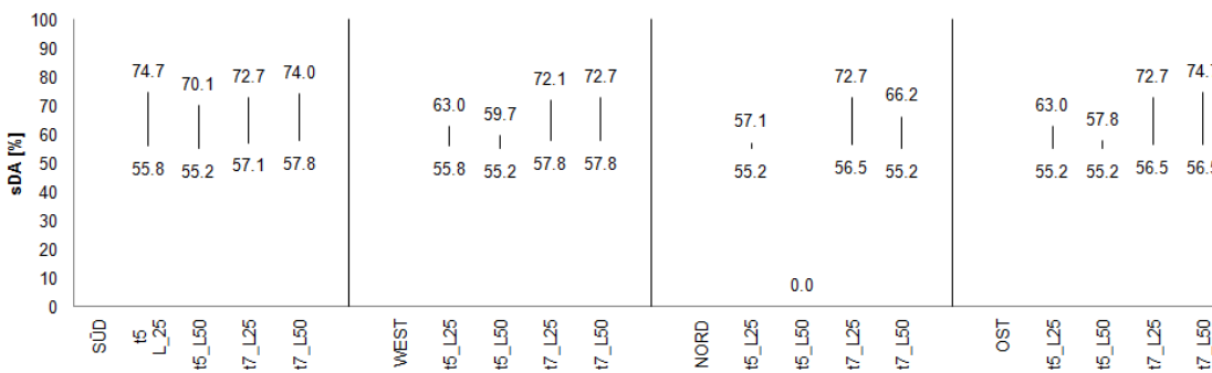
Abbildung 13_Boxplot Ergebnis sDA [%] (Eigene Darstellung: Therm. Simulation)
