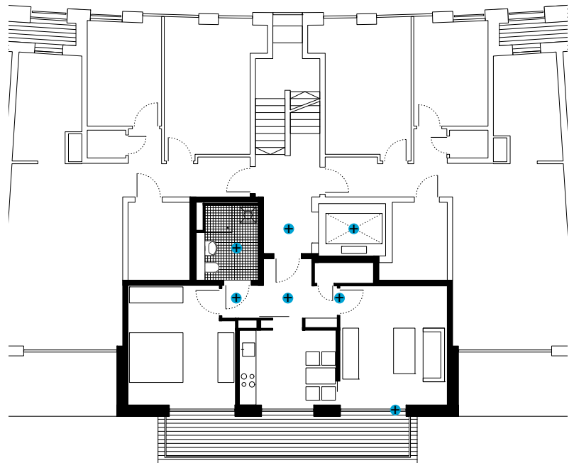
Grundriss Wohnung M 1:200
