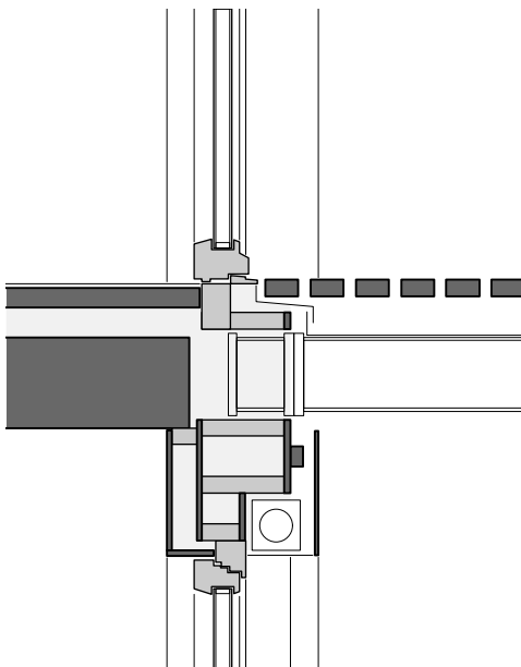
39 Detail Balkonschwelle M 1:20
