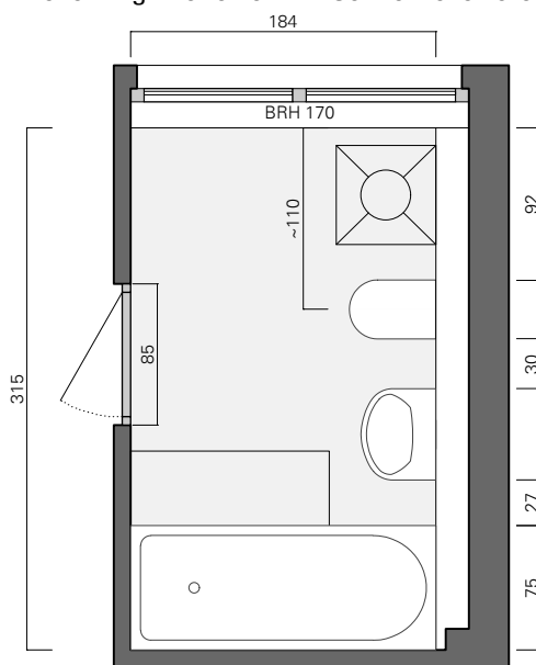
62 Grundriss Bad M 1:50
