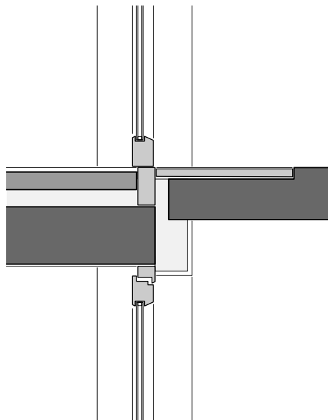
64 Detail Wohnungstür M 1:20
