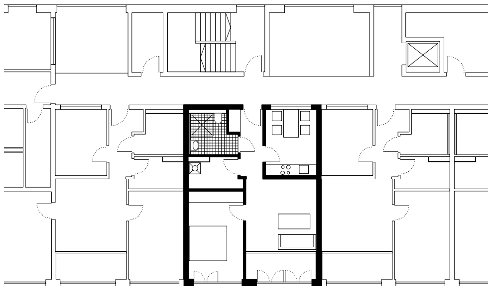
67 Grundriss Whg. M 1:200
