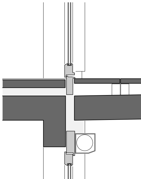
45 Detail Balkonschwelle M 1:20
