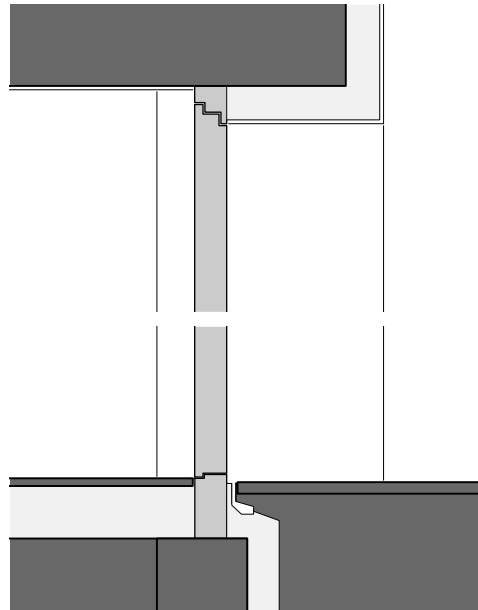
52 Detail Hauseingang M 1:20
