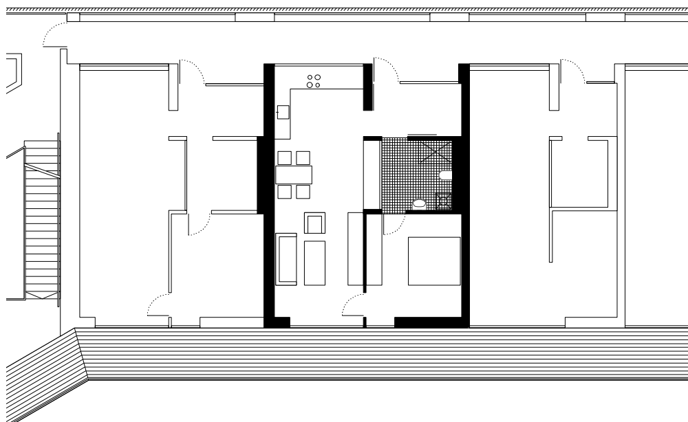
83 Grundriss Whg. M 1:200
