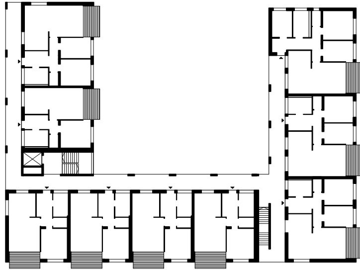
60 Grundriss RG M 1:500
