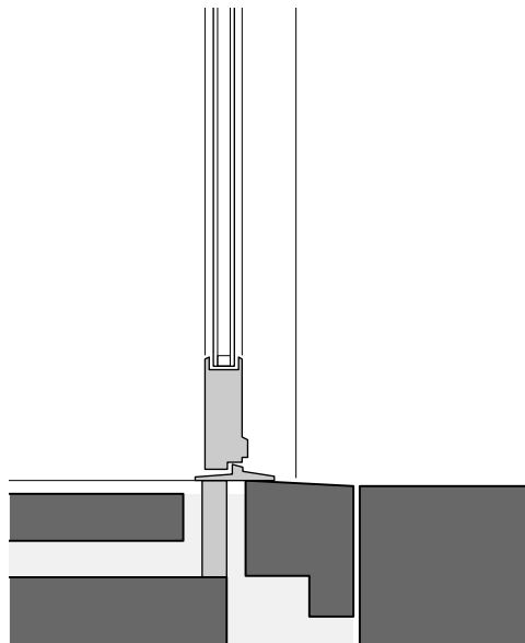
90 Detail Schwelle M 1:10
