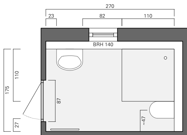
20 Grundriss Bad M1:50
