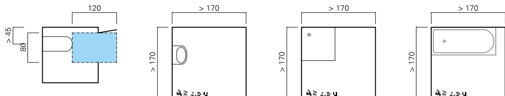
Abb. 25 Anpassbarer Bad-/Duschraum nach SIA 500:2009, 10.2.1 Schweizer Anforderungen an Nutz- und Bewegungsflächen für das hindernisfreie WC, bzw. Bad s.u.
