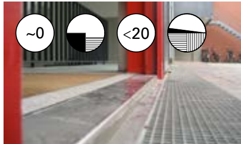
Hauseingang (Perspektive)
