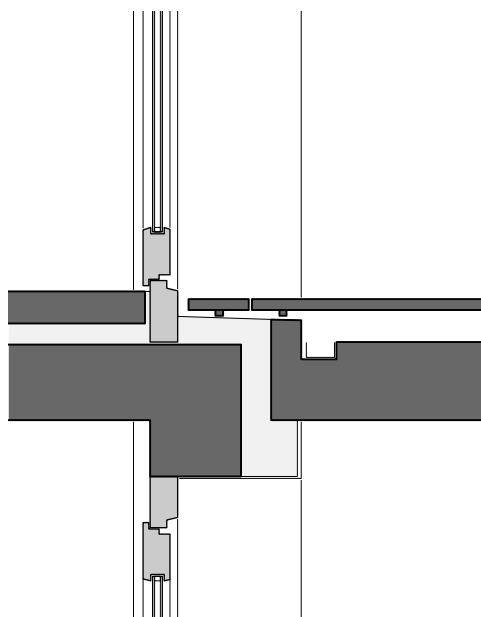
51 Detail Balkon M 1:20
