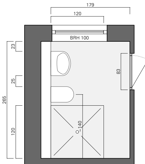
44 Grundriss Bad M 1:50
