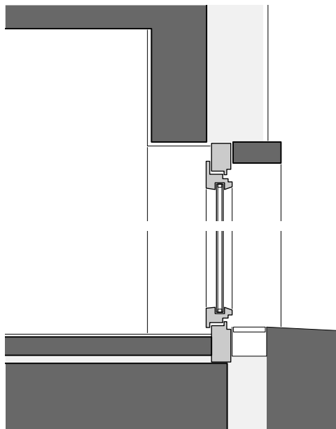
69 Detail Terrasse M 1:20
