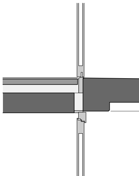
58 Detail Wohnungseingang 1:20
