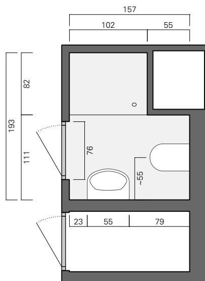
4 Grundriss Bad M 1:50
