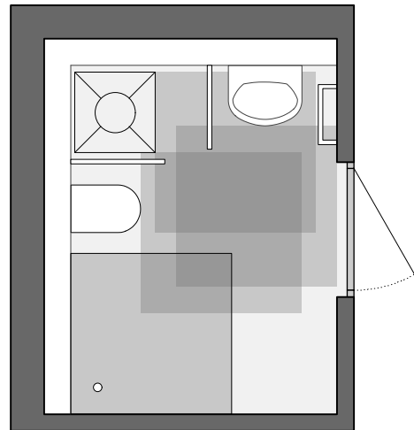
02 2,00* x 2,61* = 5,3 m 2
