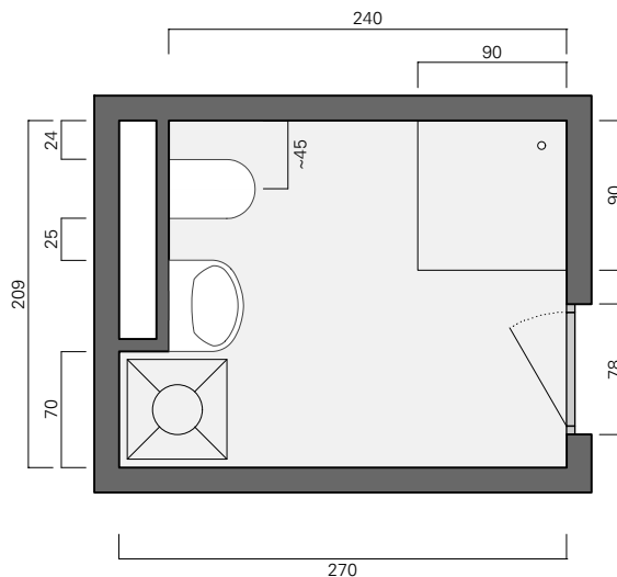
50 Grundriss (Dusch-)Bad M 1:50
