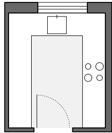
04 Fläche 7,7 m 2
