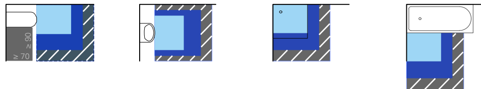
Abb. 6 Bewegungsflächen vor Sanitäröbekten nach DIN 18022:1989-11, DIN 18025:1992-12, bzw. DIN 18040:2011-09 Deutsche Planungsgrundlagen nach DIN 18022 (hellblau) und Anforderungen an Einrichtungen und Bewegungsflächen nach DIN 18025-2, bzw. 18040-2 barrierefrei (dunkelblau) und rollstuhlgerecht (schwarz)
