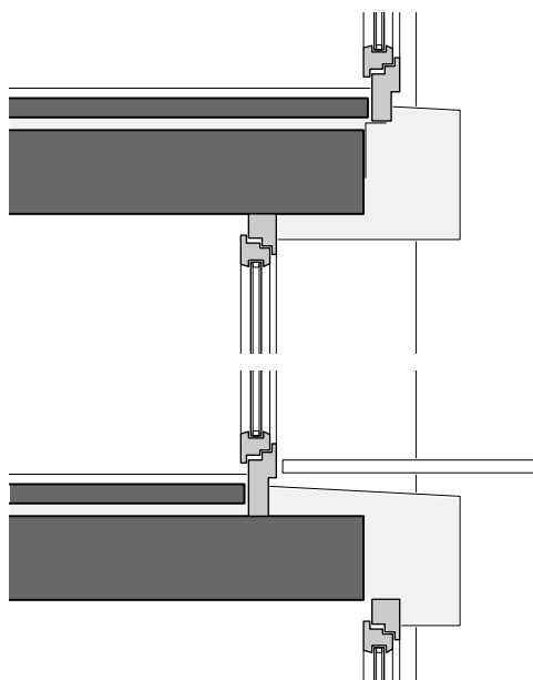
5 Detail Balkonschwelle M 1:20
