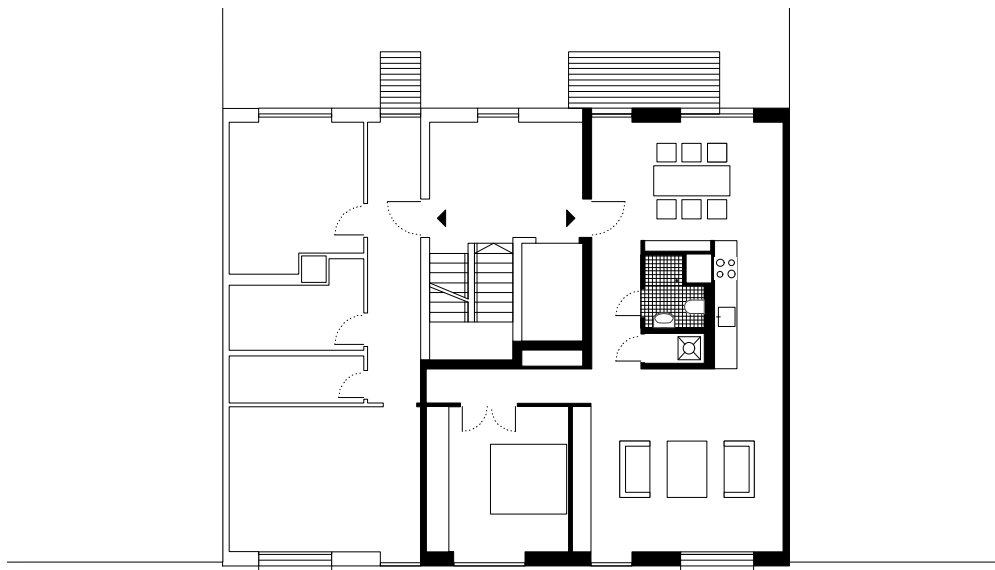
3 Grundriss Whg. M 1:200
