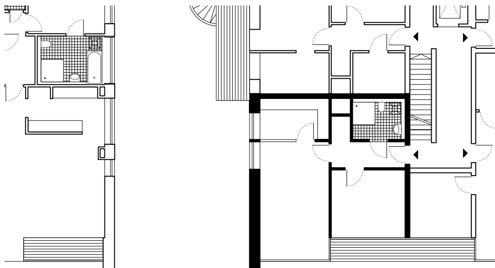
8 Grundriss Whg. M 1:200
