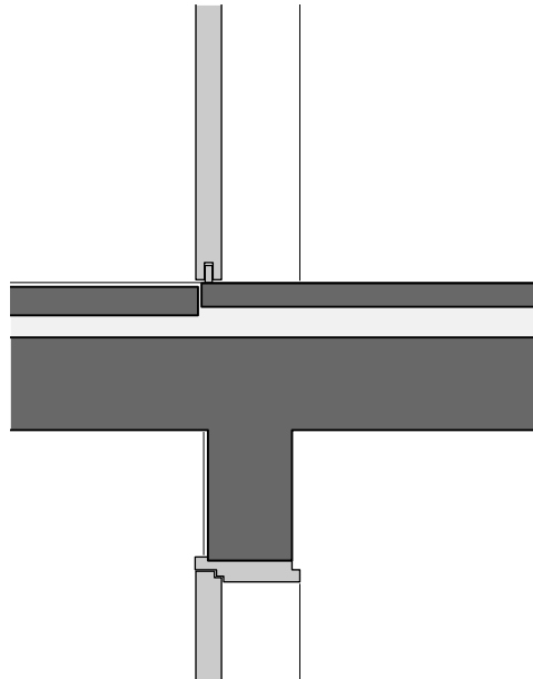
40 Detail Wohnungseingang Innenflur M 1:20
