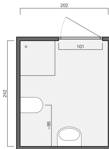
89 Grundriss Bad M 1:50
