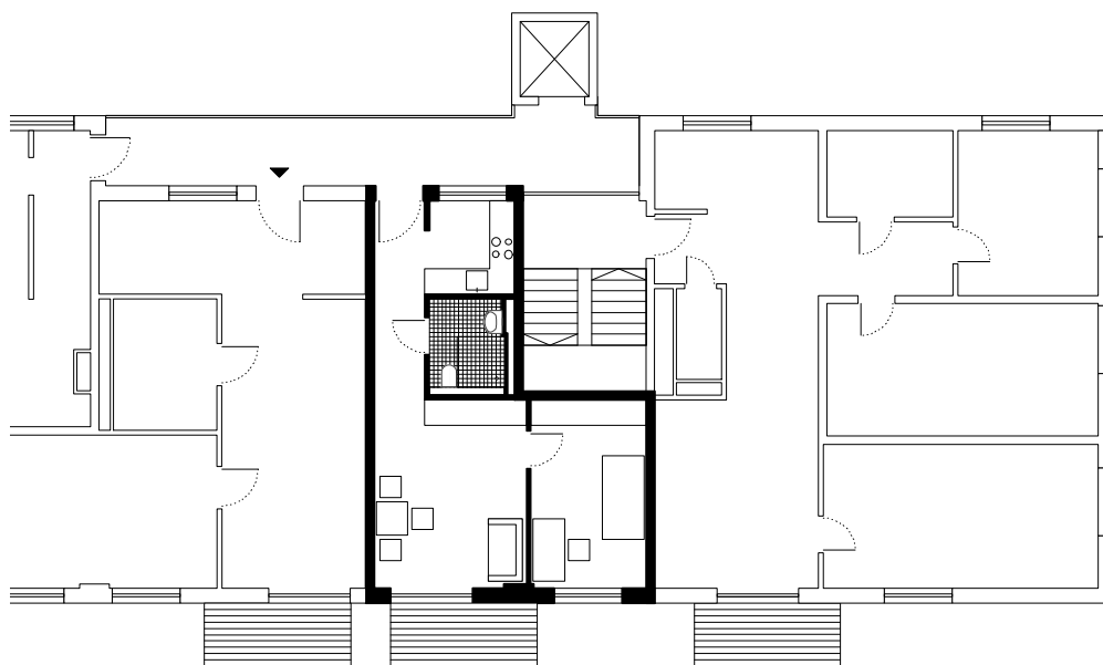
37 Grundriss Whg. M 1:200
