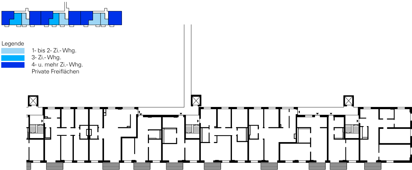
36 Grundriss RG M 1:500
