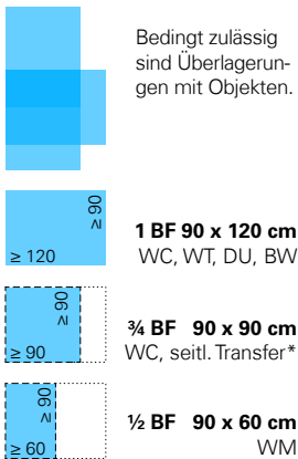
Abb. 10 Unterfahrbarkeit WT
