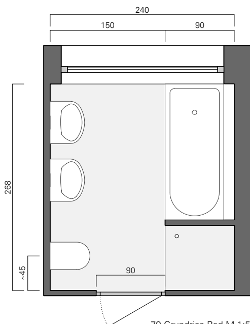
79 Grundriss Bad M 1:50
