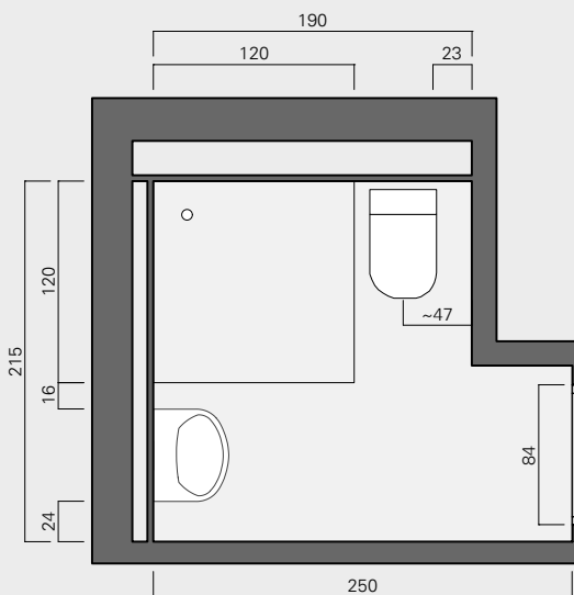
Grundriss Bad M 1:50
