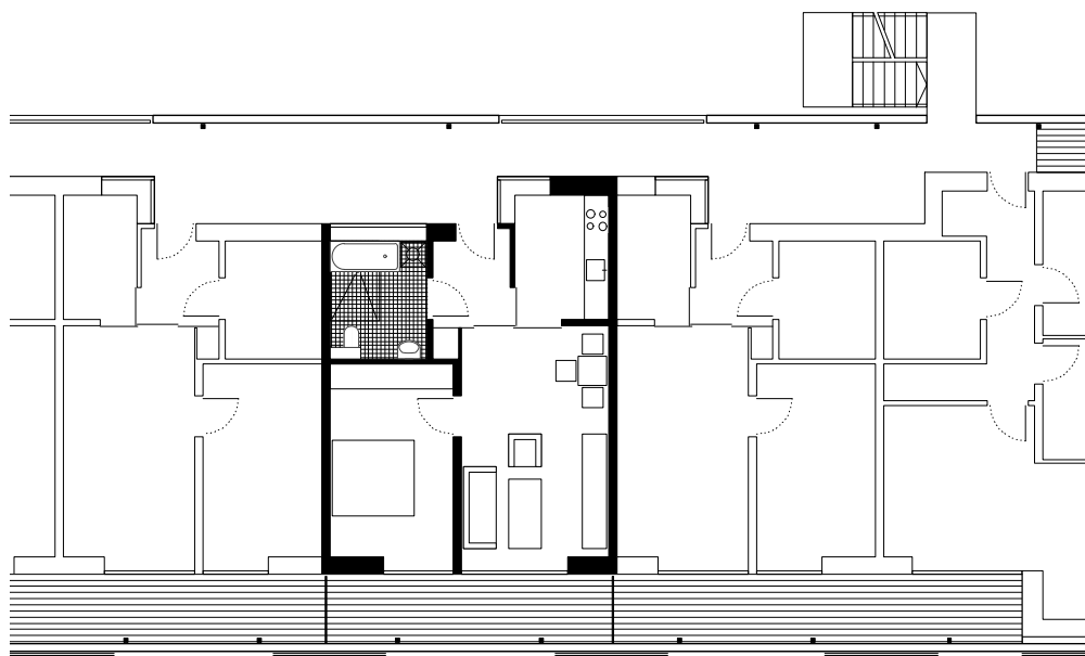
55 Grundriss Whg. M 1:200
