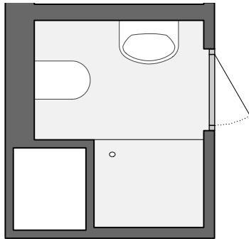
01 1,57 x 1,11 (1,93) = 2,6 m 2
