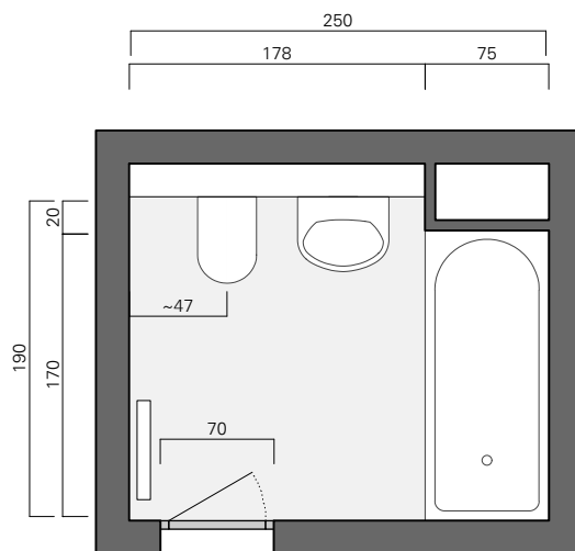
Grundriss Bad M 1:50
