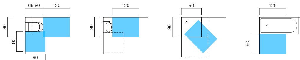
Abb. 8 Mindestanforderungen an Bewegungsflächen für das barrierefrei anpassbare und vorbereitete Bad (ready) Für jedes barrierefrei anpassbare Bad müssen drei räumliche Regeln realisiert, d.h. kombiniert werden, nachweislich für jede Einrichtung die jeweilige Bewegungsfläche, die minimale Nutzfläche sowie eine bestimmte Dreh- und Wendefläche. Hier dargestellt ist die Erste von diesen drei Regeln.
