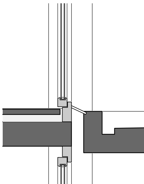
16 Detail Balkonschwelle M 1:20
