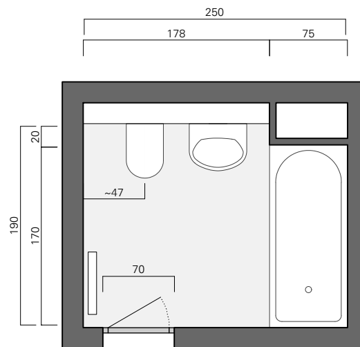
26 Grundriss Bad M 1:50
