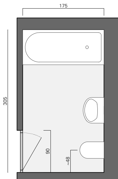
75 Grundriss Bad M 1:50
