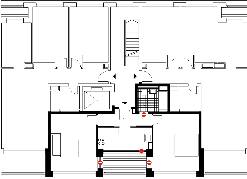
Grundriss Wohnung M 1:200
