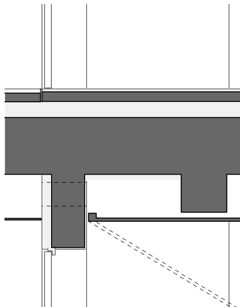
34 Detail Wohnungseingang M 1:20
