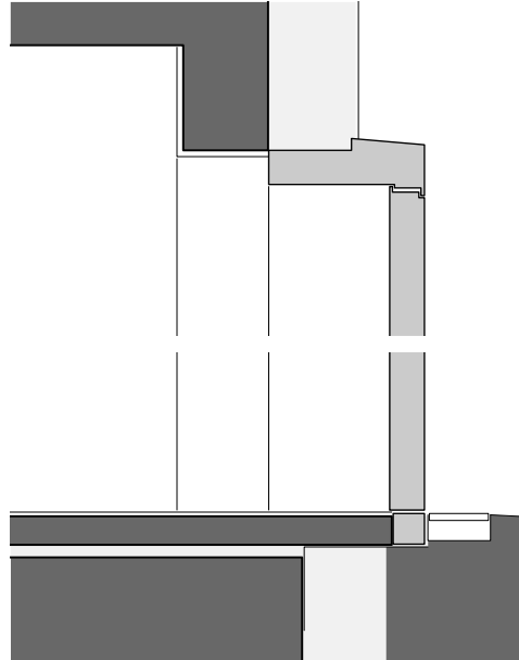
70 Detail Eingang M 1:20
