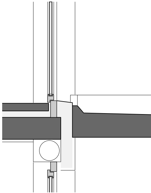
21 Detail Balkonschwelle M 1:20
