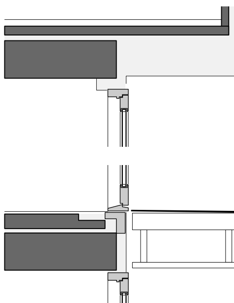
91 Detail Balkontür M 1:20
