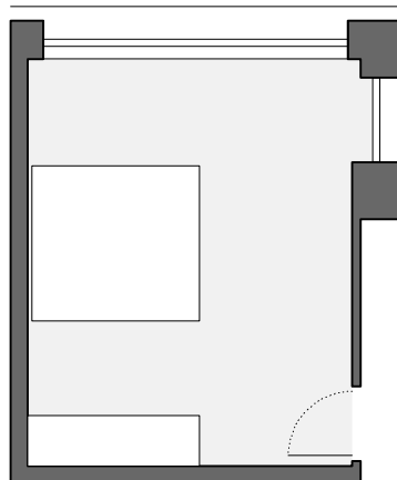
05 Fläche 18,9 m 2
