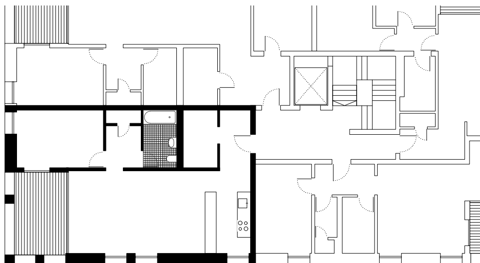
74 Grundriss Whg. M 1:200
