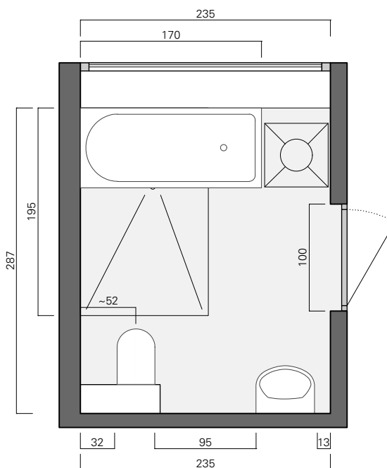
56 Grundriss Bad M 1:50
