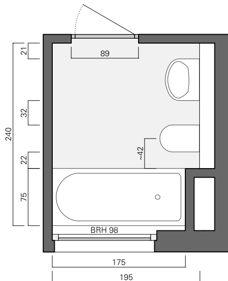
15 Grundriss Bad M 1:50
