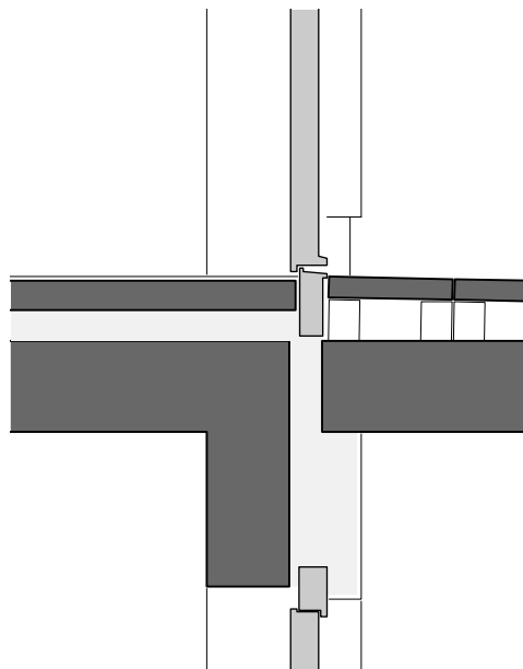
46 Detail Wohnungseingang M 1:20
