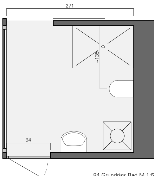
84 Grundriss Bad M 1:50
