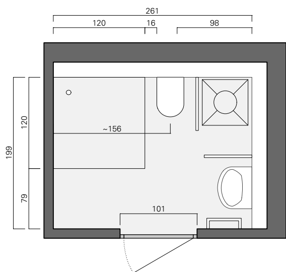
9 Grundriss Bad M 1:50
