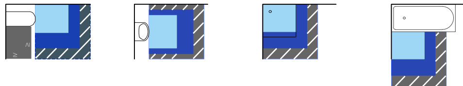
Abb. 24 Bewegungsflächen vor Sanitäröbekten nach DIN 18022:1989-11, DIN 18025:1992-12, bzw. DIN 18040:2011-09 Deutsche Planungsgrundlagen nach DIN 18022 (hellblau) und Anforderungen an Einrichtungen und Bewegungsflächen nach DIN 18025-2, bzw. 18040-2 barrierefrei (dunkelblau) und rollstuhlgerecht (schwarz)
