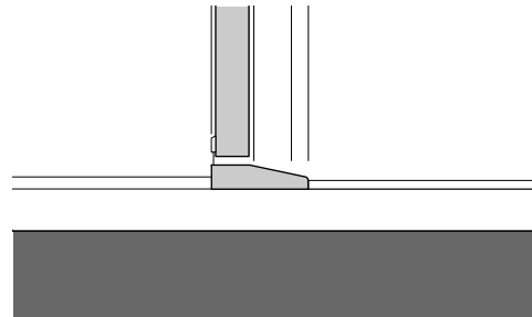
80 Detail Schwelle entsprechend ISO 21542 M 1:10
