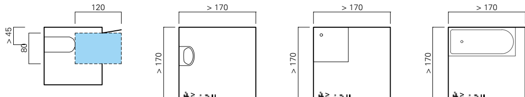
Abb. 7 Anpassbarer Bad-/Duschraum nach SIA 500:2009, 10.2.1 Schweizer Anforderungen an Nutz- und Bewegungsflächen für das hindernisfreie WC bzw. Bad
