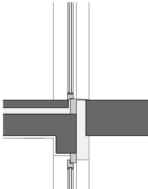
22 Detail Wohnungseingang M 1:20
