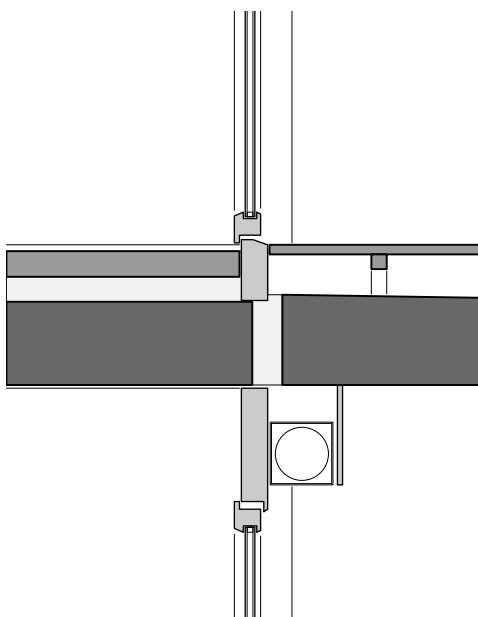
63 Detail Balkon M 1:20
