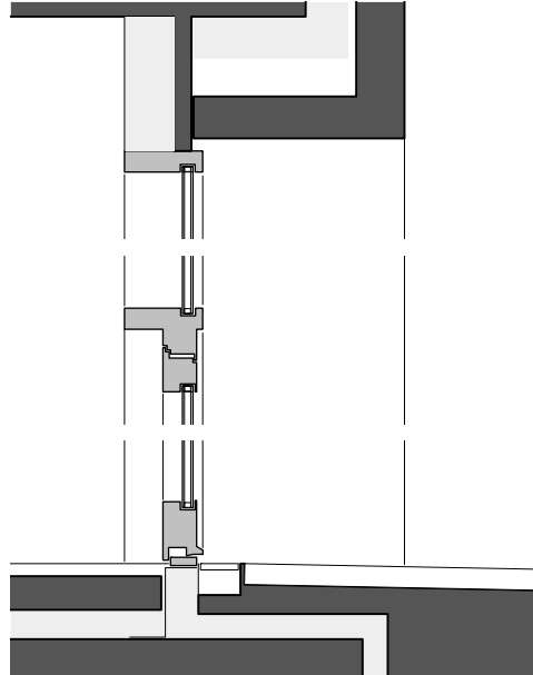
11 Detail Eingang M 1:20
