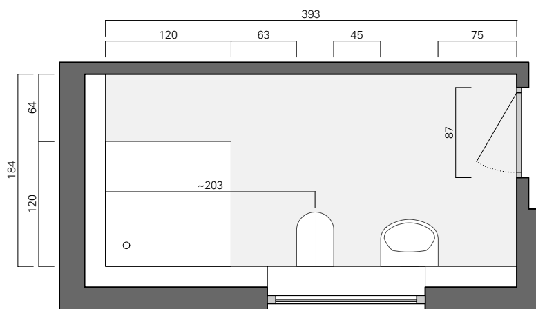
32 Grundriss Bad M 1:50
