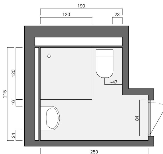
68 Grundriss Bad M 1:50
